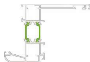
Dormant RENOVATION avec aile de 60 mm
