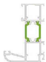
Dormant NEUF sans aile pour pose en tunnel
