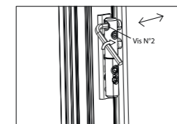
Réglage en largeur
