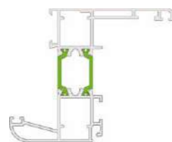
Dormant RENOVATION avec aile de 40 mm
