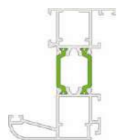
Dormant NEUF avec aile de 9 mm
