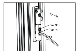
Réglage de la compression
